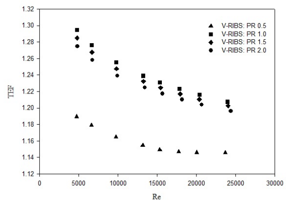
รูปที่ 7. ความสัมพันธ์ระหว่าง TEF กับ Re
