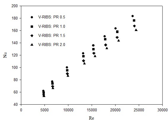
รูปที่ 3. ความสัมพันธ์ระหว่าง Nu กับ Re
