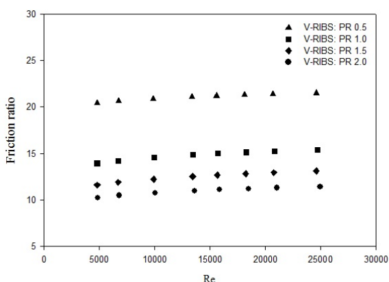
รูปที่ 6. ความสัมพันธ์ระหว่าง f/f_0 กับ Re
