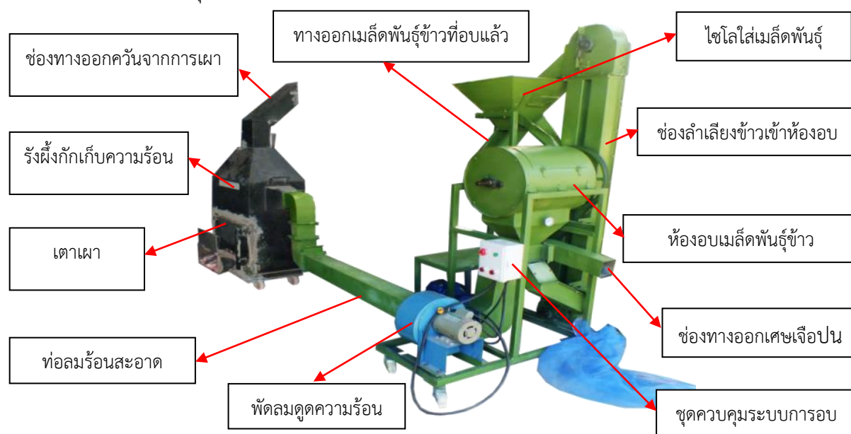
ภาพที่ 7 เตาเผาแบบรังผึ้งกักเก็บความร้อนสำหรับอบเมล็ดข้าวพื้นเมืองพันธุ์ปะกาอำปี้ล
