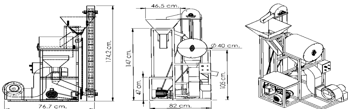
ภาพที่ 5 แบบตู้อบและคัดแยกเมล็ดพันธุ์ข้าวพื้นเมือง
